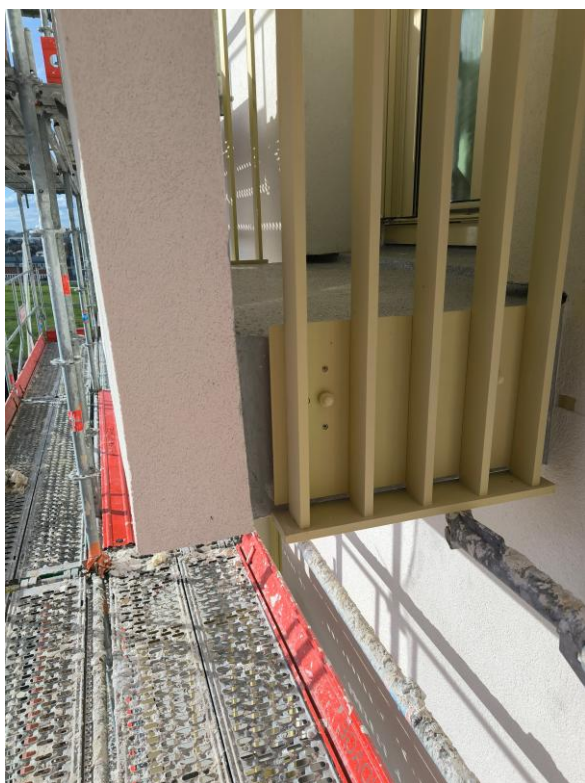
Figure 15 Sous face de balcon au 8 e étage (façade nord)
