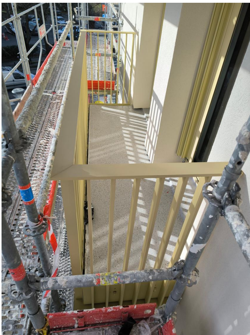
Figure 3 Garde-corps au 3e étage
